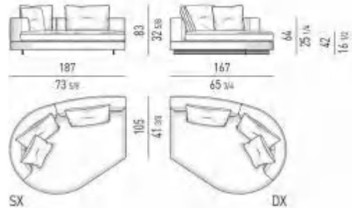
CHAISE-LONGUE RAY - LOW CM 187x167 CHAISE-LONGUE RAY - LOW CM 187x167
