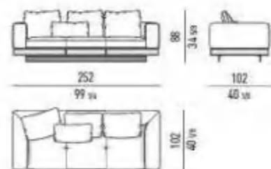
DIVANO CM 252 SOFA CM 252
