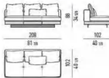
ELEMENTO CENTRALE CM 208 CENTRAL ELEMENT CM 208
