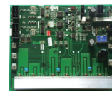
MIPCB71
