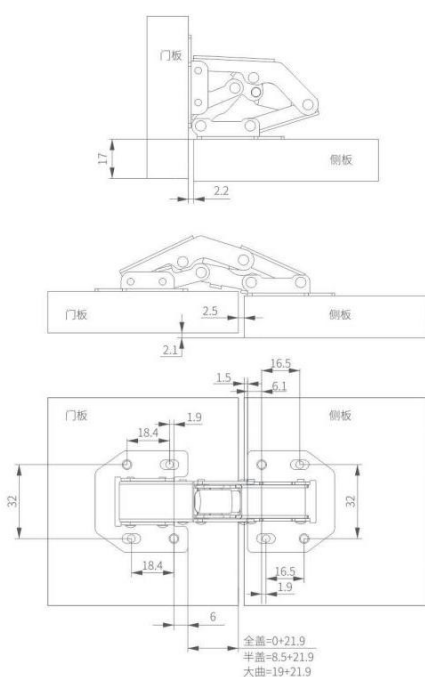
安装小盖位(反)
