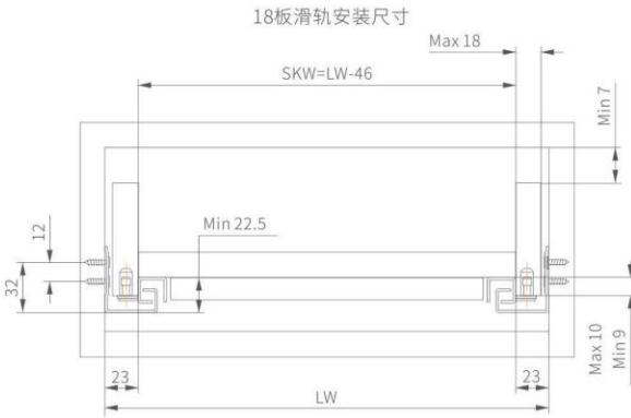
18板滑轨安装尺寸
