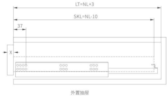
外置抽屉
