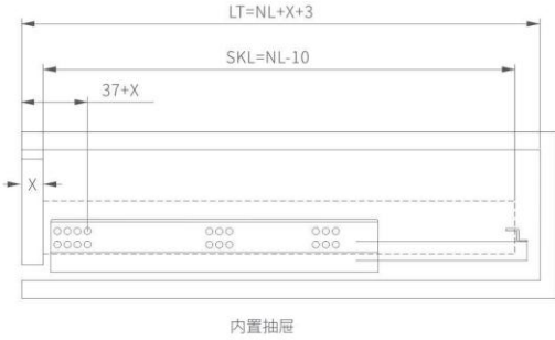
内置抽屉
