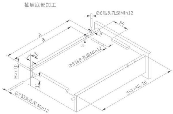
抽屉底部加工
