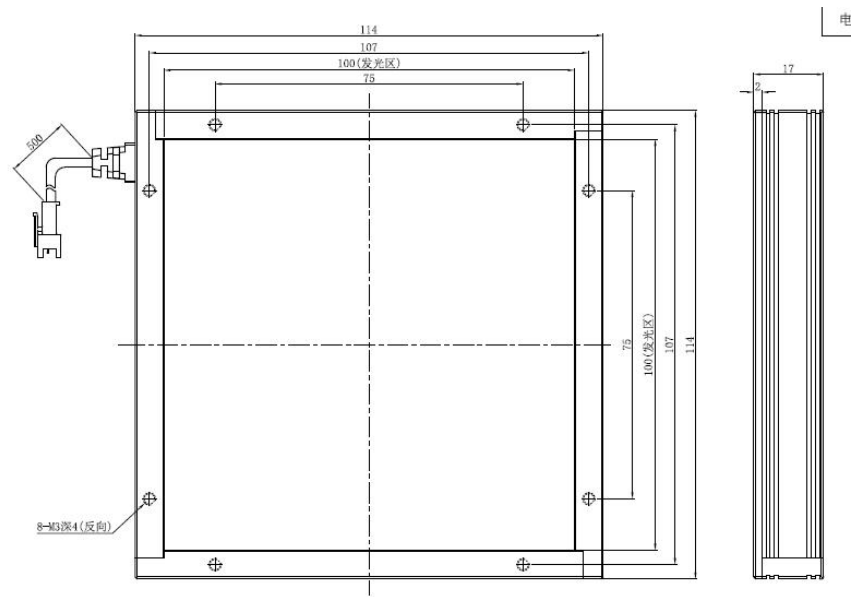
产品尺寸图
