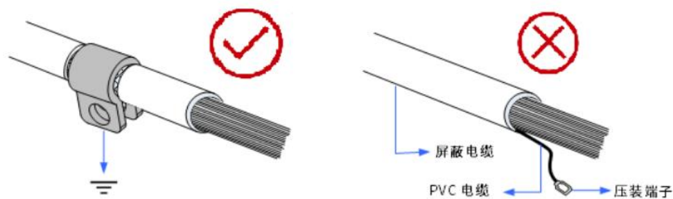
屏蔽线缆接地要求示意图 1
