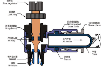
出气节流阀 /Air outlet controller
