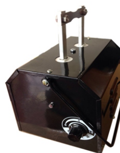
WJ511-3 手动切嘴机 MANUAL POULTRY DEBEAKER
